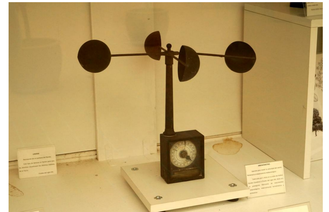
Anemómetro. Fabricado por J. Hicks en su taller de Hatton Garden (Londres) a finales del siglo XIX. Hicks era un prestigioso fabricante de instrumentos meteorológicos, especialmente termómetros y barómetros.
